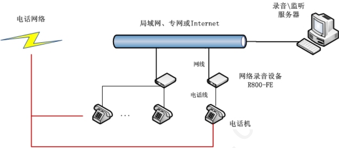
录音系统分布式网络结构图
